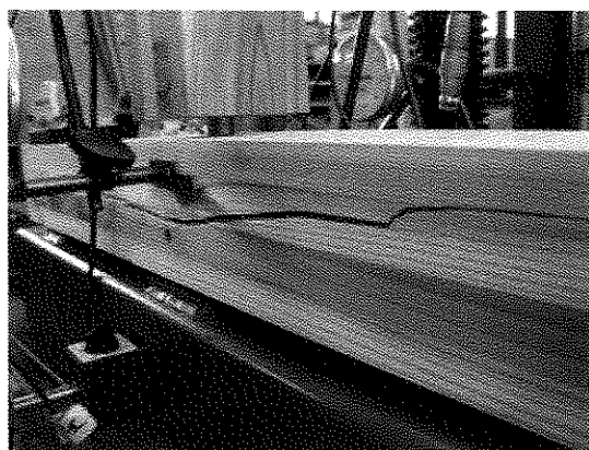
【②梁の横引張破壊】
