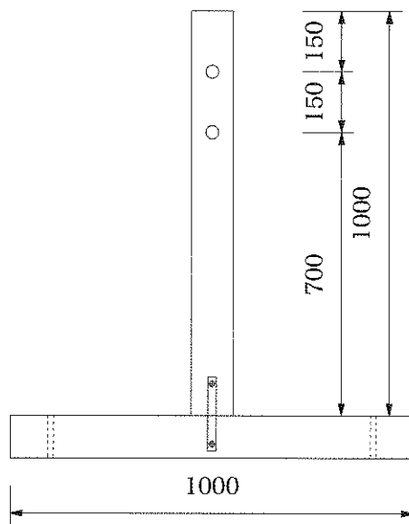
図 1 引張試験体
