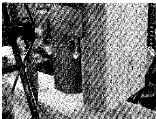
【③柱のせん断破壊】
