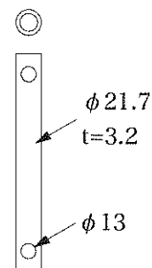
図 2 接合金物（材質：SS400）
