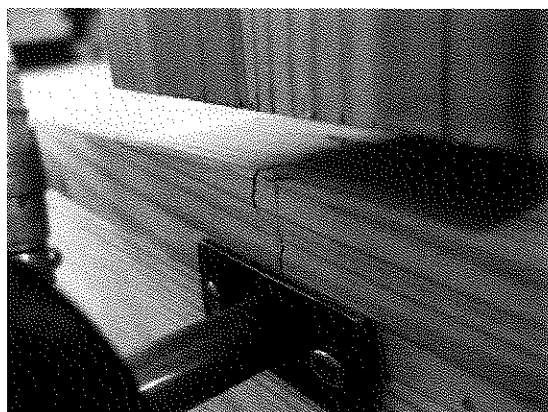
【①ドリフトピンから生じた割裂破壊】
